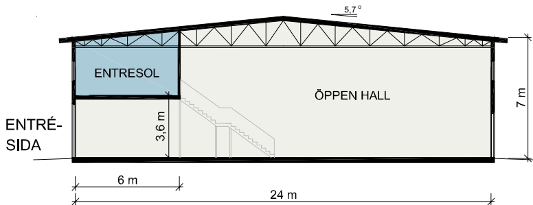
PRINCIPSEKTION A 1:300
