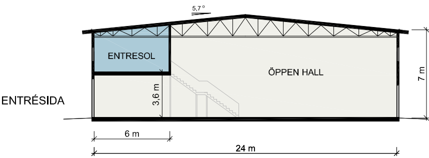
PRINCIPSEKTION A 1:300
